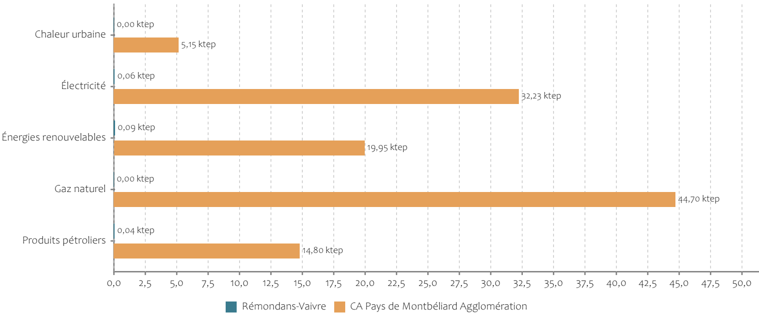
Consommations du secteur résidentiel par type d'énergie
